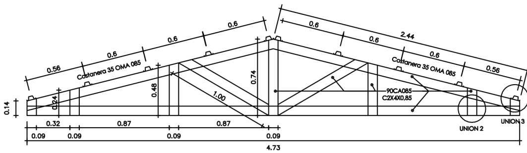
CERCHA TIPO 1 ————— 1:20
