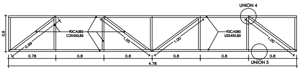
VIGA 1 ————— 1:20
