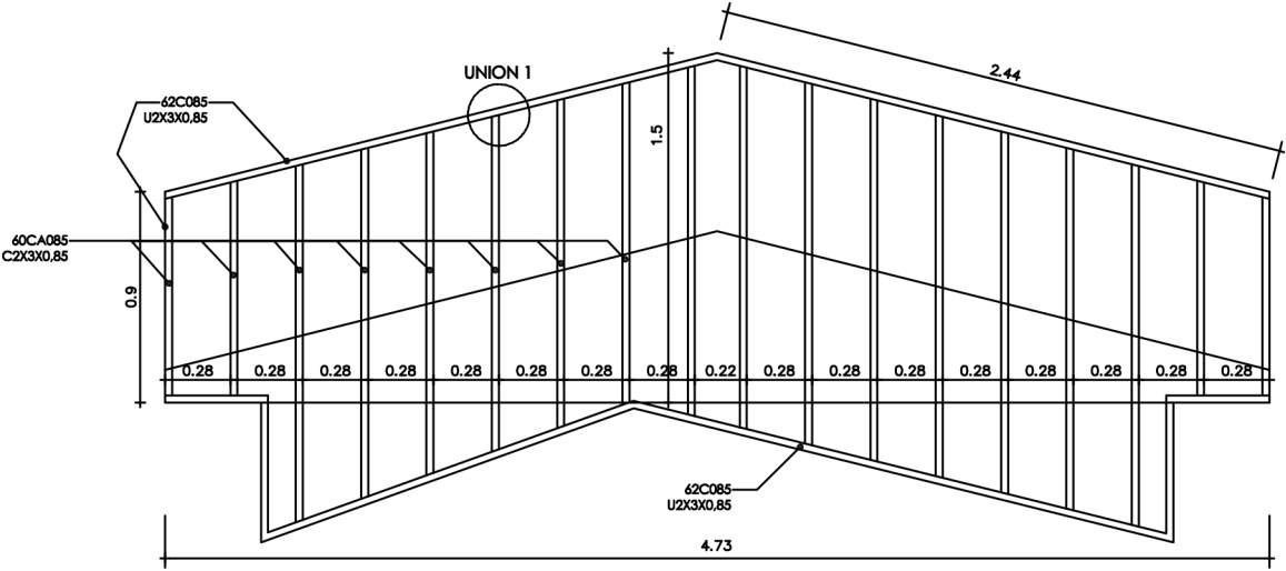
CORTAFUEGO MINVU A.2.3.120.20 ————— 1:20
