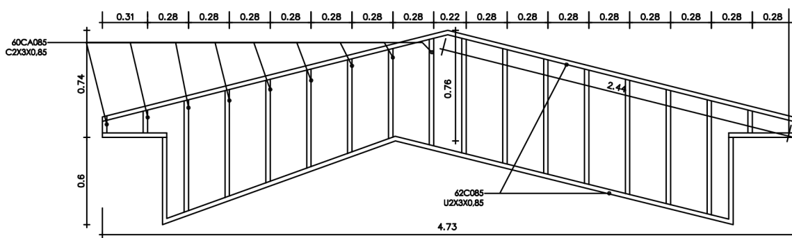
FRONTON ————— 1:20
